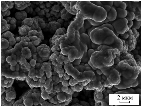
Рис. 6. Микроструктура поверхности меди, осажденной из щелочного раствора на основе пропиленгликоля, содержащего ОЭДФ
