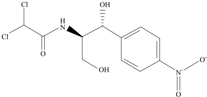
Рис. 1. Структурная формула хлорамфеникола
