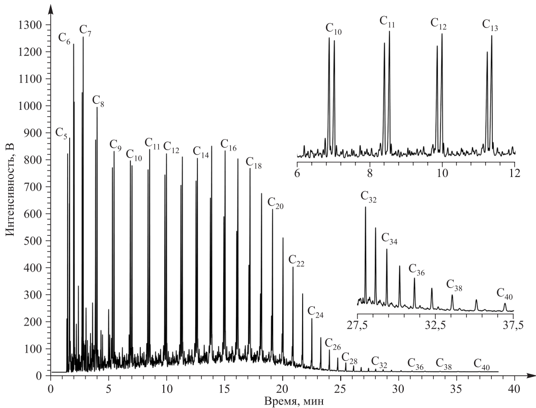
Рис. 1. Хромотограмма пиролизата ПЭ
