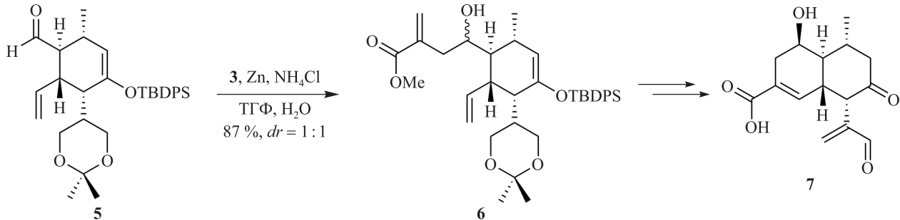
Рис. 3. Реакция аллилирования по Барбье в синтезе панала (7)
