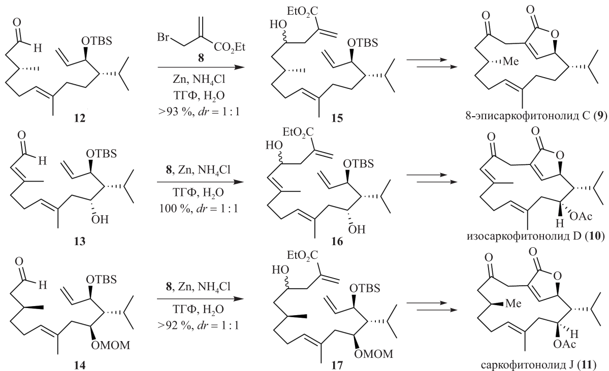
Рис. 4. Реакция аллилирования по Барбье в синтезе соединений группы саркофитенолидов (9–11)
