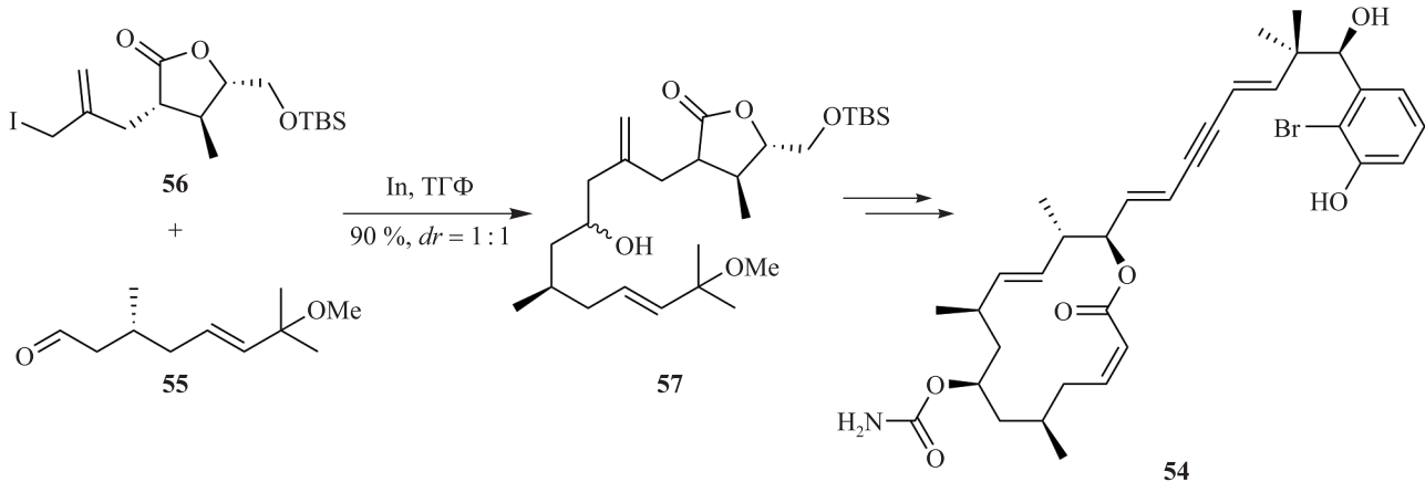
Рис. 14. Реакция аллилирования по Барбье в синтезе (–)-каллиспонгиолида (54)
