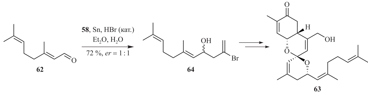
Рис. 16. Реакция аллилирования по Барбье в синтезе (–)-форбакетала А ( 63 )
