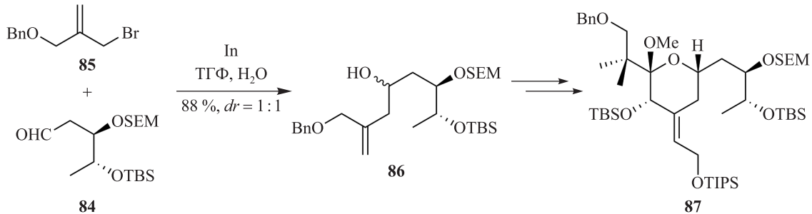
Рис. 23. Реакция аллилирования по Барбье в синтезе строительного блока бриостатинов ( 87 )
