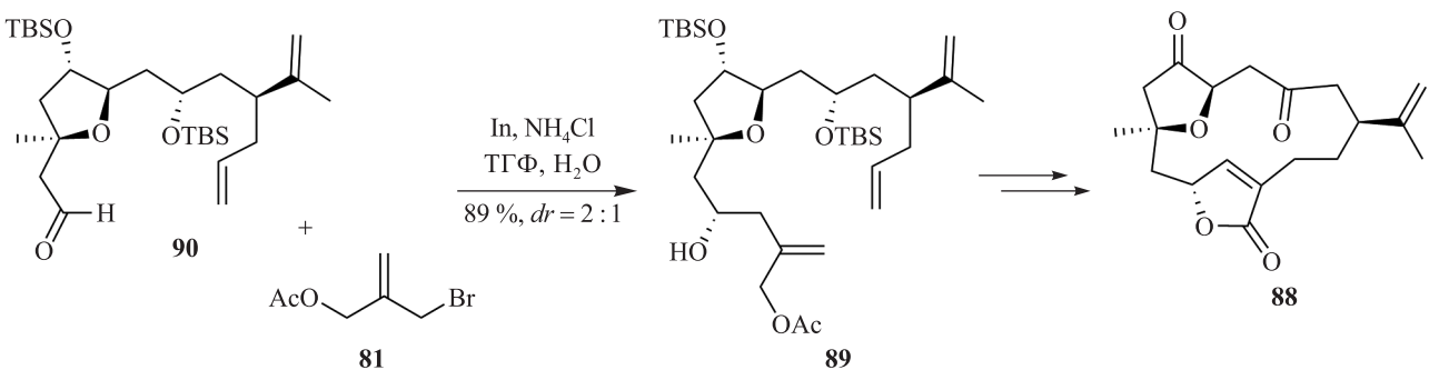
Рис. 24. Реакция аллилирования по Барбье в полном синтезе (+)-10-эпигиросанолида E ( 88 )
