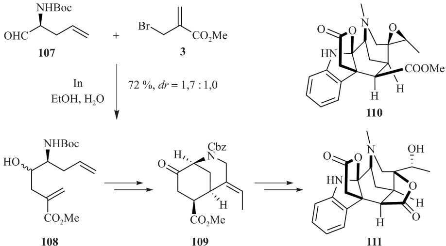
Рис. 28. Реакция аллилирования по Барбье в синтезе сколарисина К ( 110 ) и алстолактина А ( 111 )
