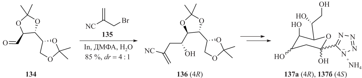
Рис. 33. Реакция аллилирования по Барбье в синтезе производных сиаловой кислоты ( 137a и 1376 )
