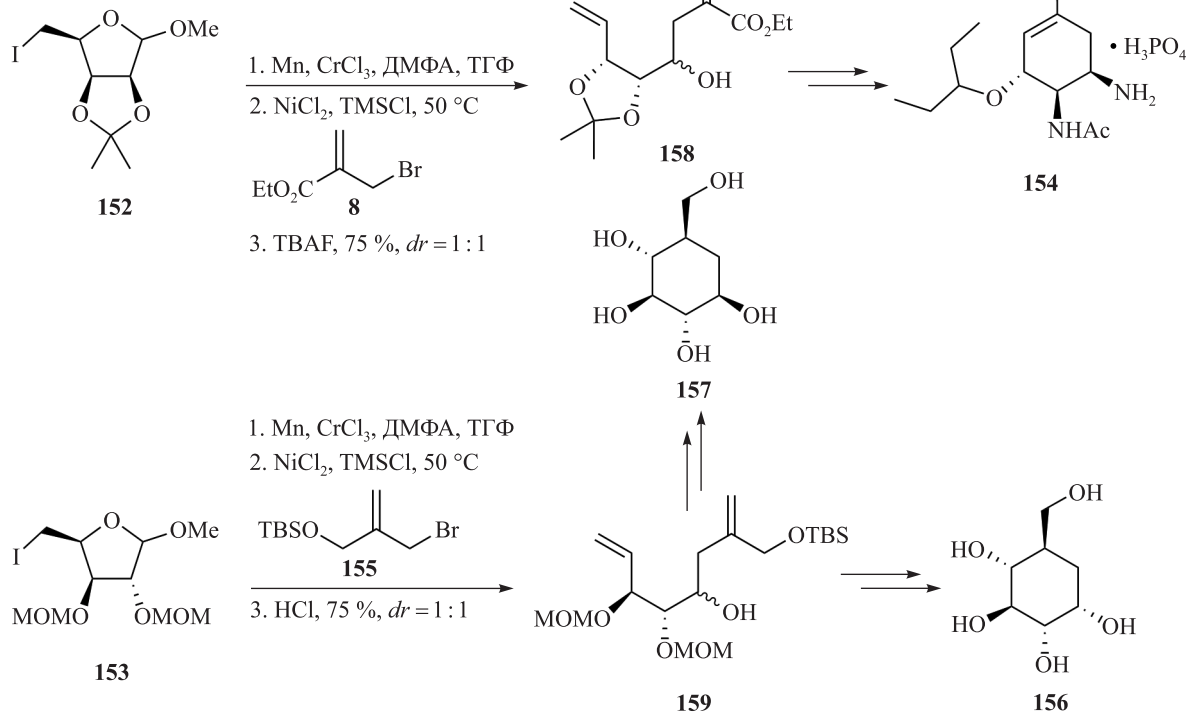
Рис. 35. Реакция Нозаки – Хиямы – Киши в синтезе карбосахаров с глюкозидазной ингибирующей активностью ( 154 , 156 и 157 )
