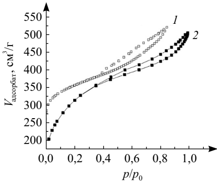
Рис. 4. Изотермы низкотемпературной адсорбции азота на АУ: 1 – ОУ-А + 8 % Na-CAЦ; 2 – АС + 8 % Na-CAЦ
