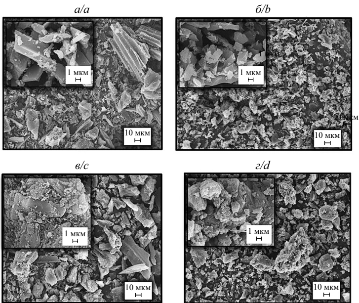
Рис. 5. СЭМ-изображение АУ:
