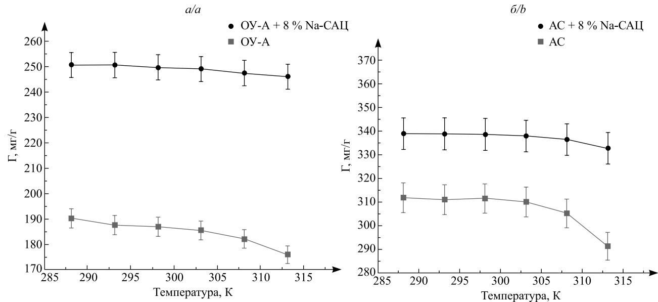
Рис. 7. Зависимость удельной адсорбции ЦЕФОТ на АУ от температуры для исходных и модифицированных ОУ-А (а) и АС (б)
