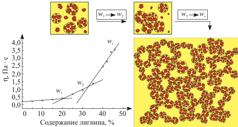
Рис. 3. Зависимость вязкости дисперсий ГЛ в ИМ от содержания ГЛ и схематичное изображение процесса структурообразования
