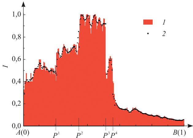
Рис. 6. Распределение интенсивности ( I ) красного цвета вдоль диагонали AB на микрофотографии до (1) и после (2) трассировки
