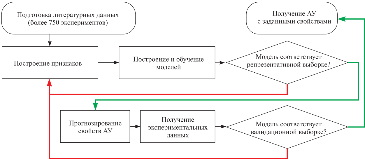
Рис. 11. Схема проведения машинного обучения
