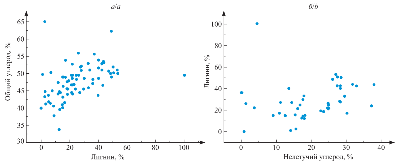
Рис. 15. Корреляционные поля: a – содержания общего углерода С и лигнина; б – содержания лигнина и нелетучего углерода
