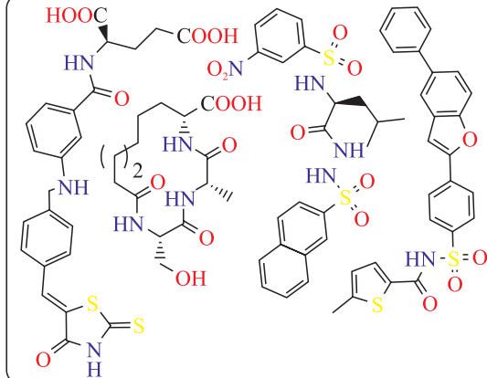
Рис. 3. Структуры некоторых известных ингибиторов белков MurA (а), MurB (б) и MurC – MurF (в)
