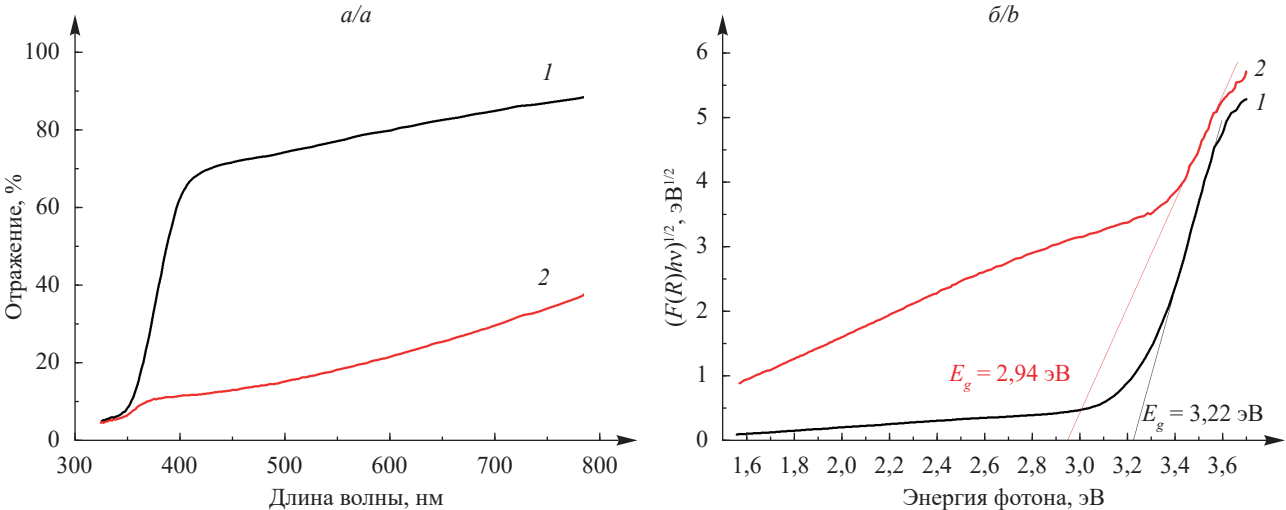
Рис. 1. Спектры диффузного отражения (а) и графики зависимости функции Кубелки – Мунка от энергии фотона (б) для оксидных материалов: 1 – исходный TiO 2 ; 2 – черный TiO 2
