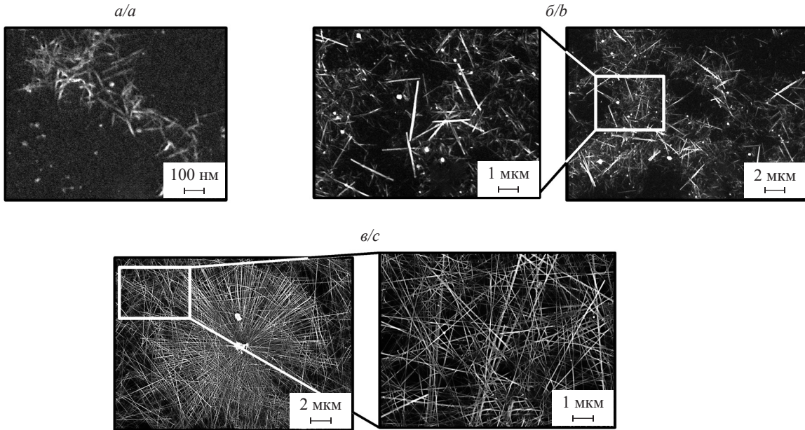
Рис. 4. Электронно-микроскопические изображения частиц 0,5\text{V}_2\text{O}_5 : 0,5\text{MoO}_3 , полученных в присутствии ПАВ I (а), ПАВ II (б), ПАВ III (в)
