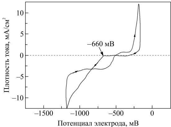
Рис. 3. Вольт-амперная кривая поляризации медного электрода в растворе, моль/л: \text{CuSO}_4 - 0,1 ; \text{NaOH} - 1,5 ; \text{C}_3\text{H}_8\text{O}_2 - 0,6 Fig. 3. Volt-ampere curve of polarisation of copper electrode in solution, mol/L: \text{CuSO}_4 - 0.1 ; \text{NaOH} - 1.5 ; \text{C}_3\text{H}_8\text{O}_2 - 0.6
