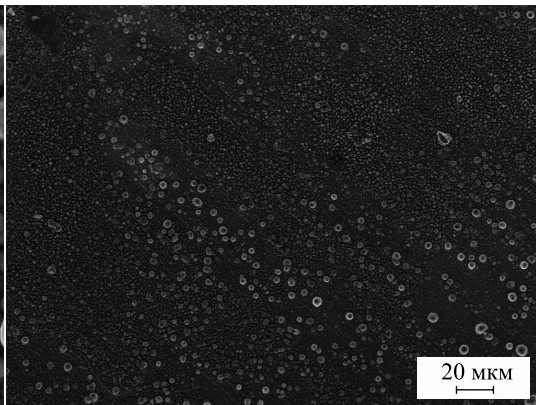
Рис. 7. Микроструктура поверхности меди, осажденной из щелочного раствора на основе пропиленгликоля, содержащего ОЭДФ и морфолин
