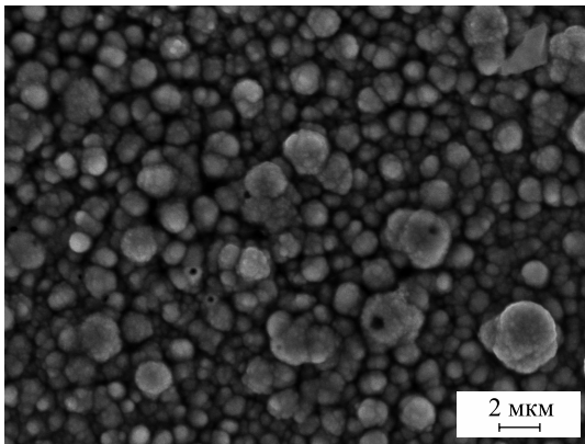
Рис. 7. Микроструктура поверхности меди, осажденной из щелочного раствора на основе пропиленгликоля, содержащего ОЭДФ и морфолин
