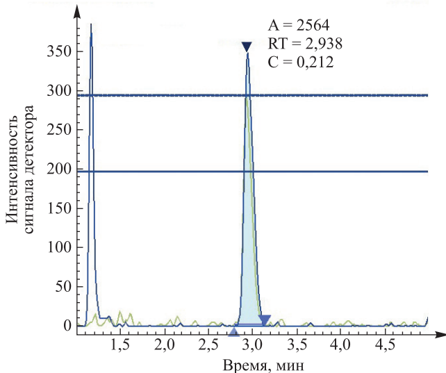
Рис. 2. Хроматограмма экстракта молочного коктейля с добавлением хлорамфеникола (A – площадь хроматографического пика; RT – время удерживания, мин; C – концентрация хлорамфеникола, мкг/кг)
