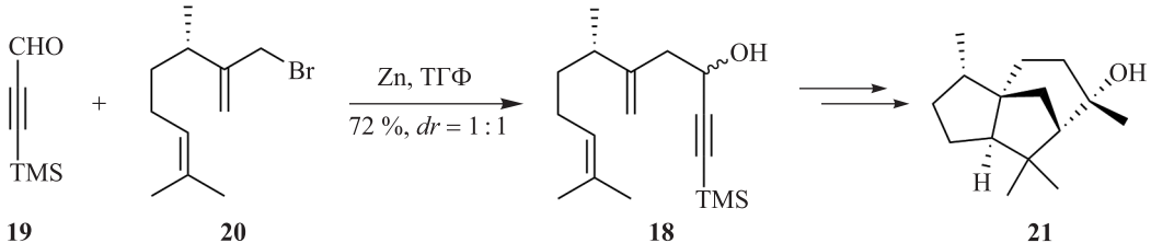
Рис. 5. Реакция аллилирования по Барбье в синтезе юниперанола ( 21 )
