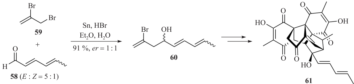
Рис. 15. Реакция аллилирования по Барбье в синтезе гомодимерицина А ( 61 )
