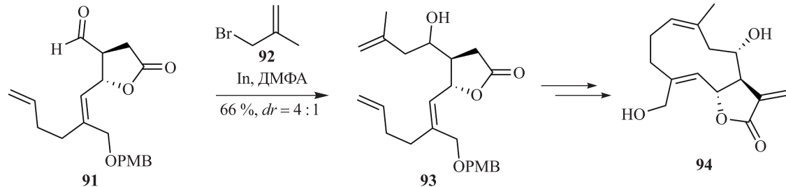
Рис. 25. Реакция аллилирования по Барбье в полном синтезе (1Z)-деациклина ( 94 )
