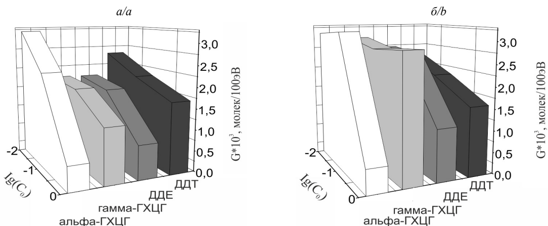
Рис. Радиационно-химический выход разложения ХОП в гексане (а) и 2-пропанол (б) после облучения в дозе 10 кГр с мощностью дозы 0,43 Гр/с
