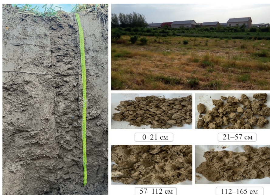
Рис. 4. Морфологические признаки разреза 3 в северо-восточном направлении Каттакурганского водохранилища
