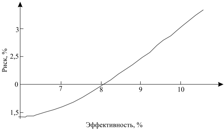
Рис. 1. Граница парето-оптимальных решений
