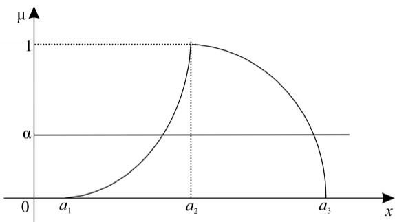
Рис. 2. Графическое представление нечеткого числа Fig. 2. The graph of a fuzzy number
