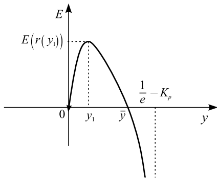
Рис. 2. График функции эластичности E = E(r(y)) для 0 < eK_p < 1 , 0 < K_p < 1
