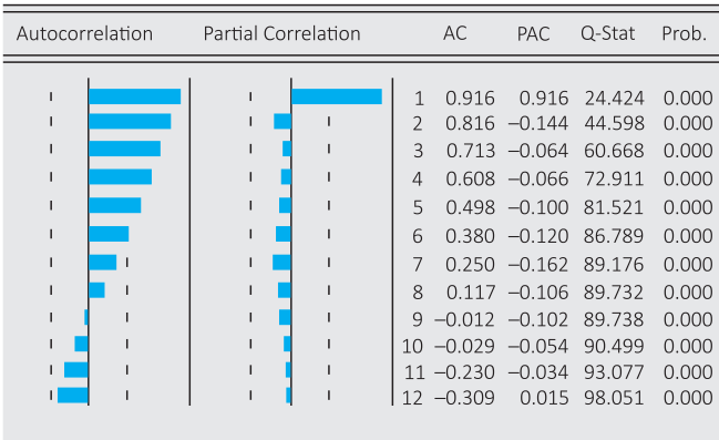
Рис. 4. Коррелограммы в уровнях (а) и в разностях (б) для ряда GDPCONST
