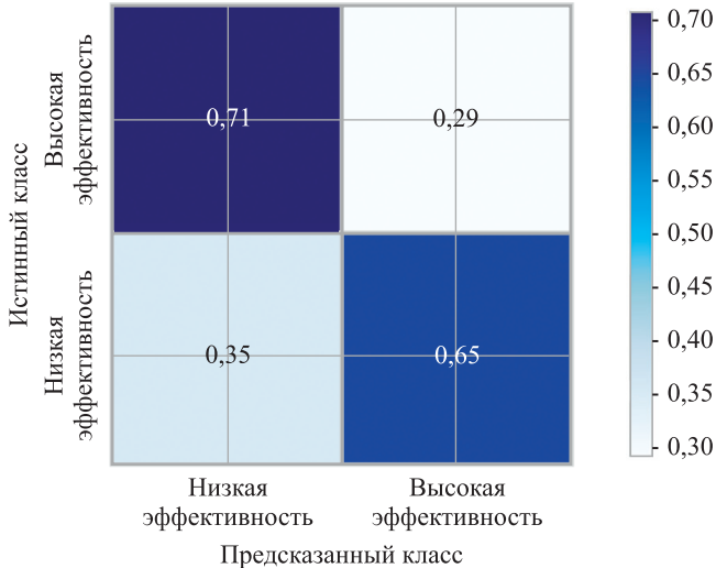
Рис. 2. Матрица ошибок модели XGBoost после постобработки порога Fig. 2. Confusion matrix of the XGBoost model after threshold post-processing
