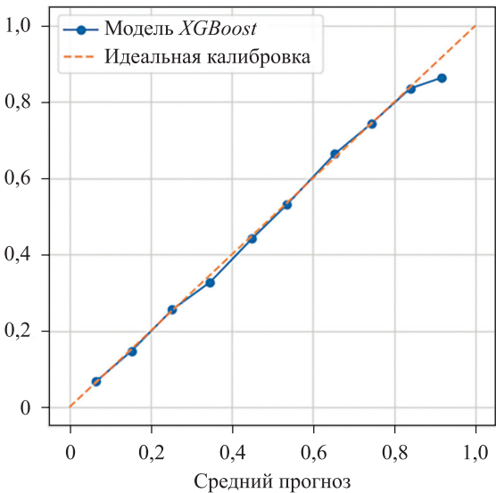
Рис. 3. Калибровочная кривая для модели XGBoost
