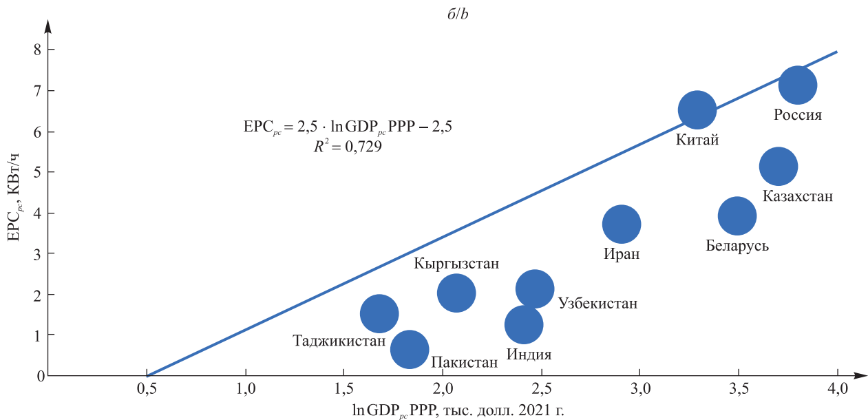
Рис. 10. Модели линейной (а) и логарифмической (б) регрессии электропотребления и GDP pc PPP Fig. 10. Models of linear (a) and logarithmic (b) regression of electricity consumption and GDP pc PPP
