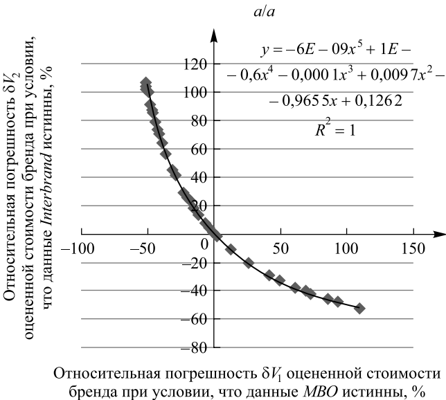
Рис. 3. Графическая интерпретация результатов исследования статистической связи исследуемых параметров \delta V_1 , \delta V_2 (a) и |\delta V_1| , |\delta V_2| (б)
