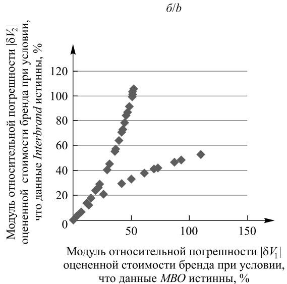
Рис. 3. Графическая интерпретация результатов исследования статистической связи исследуемых параметров \delta V_1 , \delta V_2 (a) и |\delta V_1| , |\delta V_2| (б)
