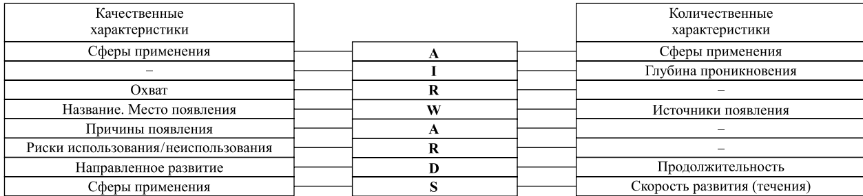
Рис. 4. Тренд-сигнал и его описание на основе модели AIRWARDS
