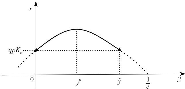
Рис. 1. График функции выручки r = r(y) для 0 < y < \frac{1}{e} - K_p , 0 < K_p < 1 , eK_p < 1
