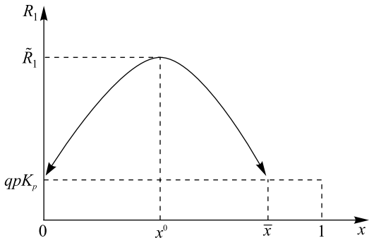
Рис. 1. График функции выручки R_1 = R_1(x) , x = k_q , в случае \frac{1-A}{AK_p} < e < \frac{1}{AK_p}
