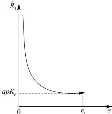
Рис. 3. График функции максимальной выручки \tilde{R}_1 = \tilde{R}_1(e) в случае 0 < e < \frac{1}{AK_p}
