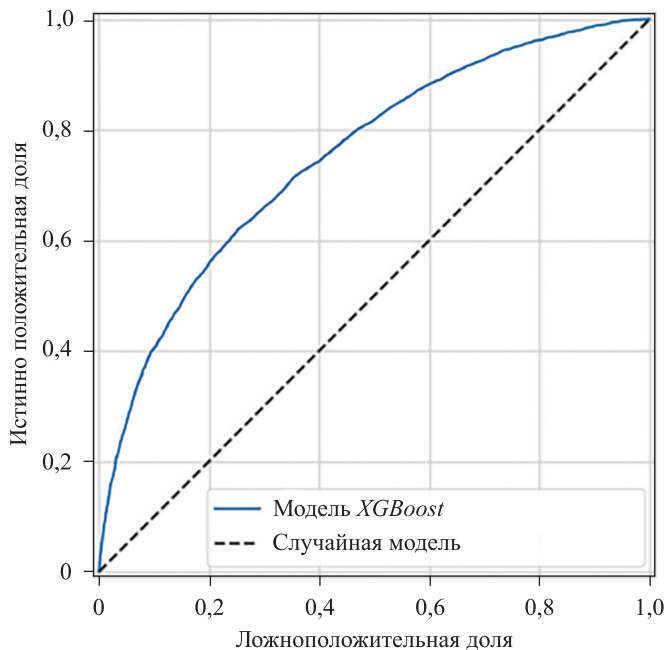
Рис. 1. ROC-кривая качества модели XGBoost (библиотека Optuna ) на тестовой выборке ( AUC = 0,75 )
