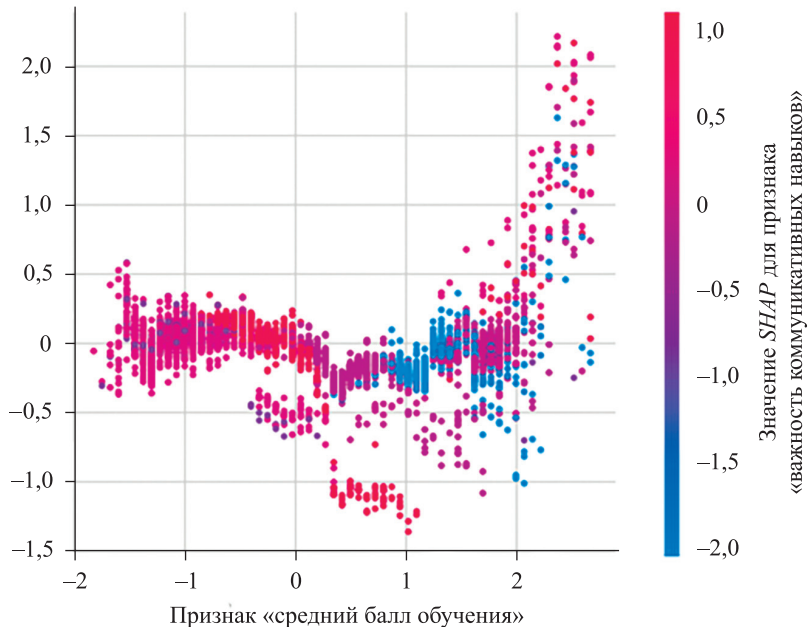
Рис. 5. Значение взаимодействия SHAP между признаками «средний балл обучения» и «важность коммуникативных навыков»
