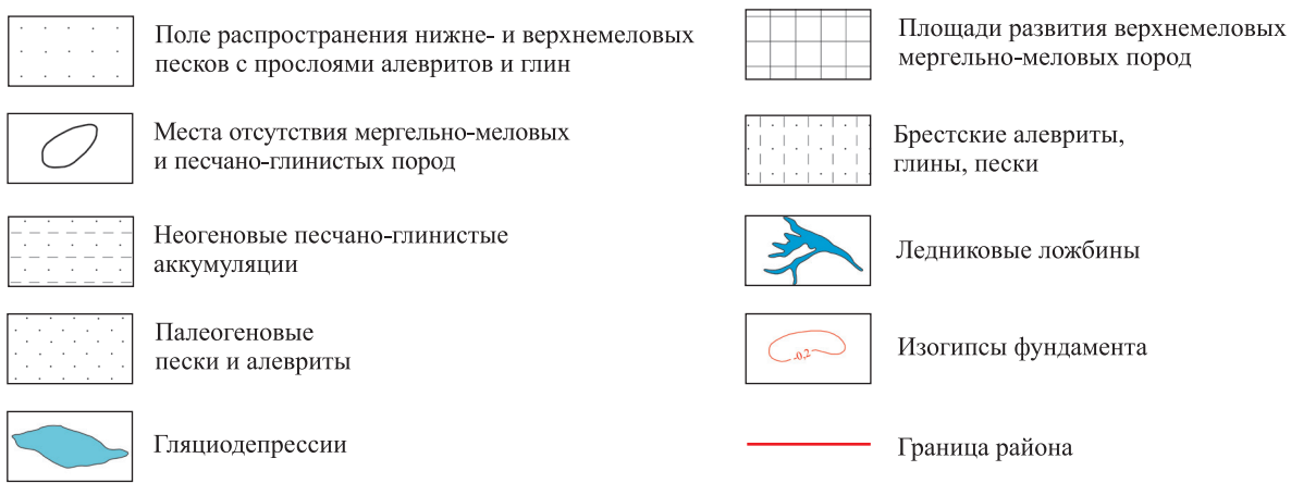
Рис. 2. Взаимосвязь ледниковых ложбин с полем развития мергельно-меловых отложений верхнего мела и песчано-глинистых образований кайнозоя и с неглубоким залеганием фундамента в пределах Белорусской антеклизы
