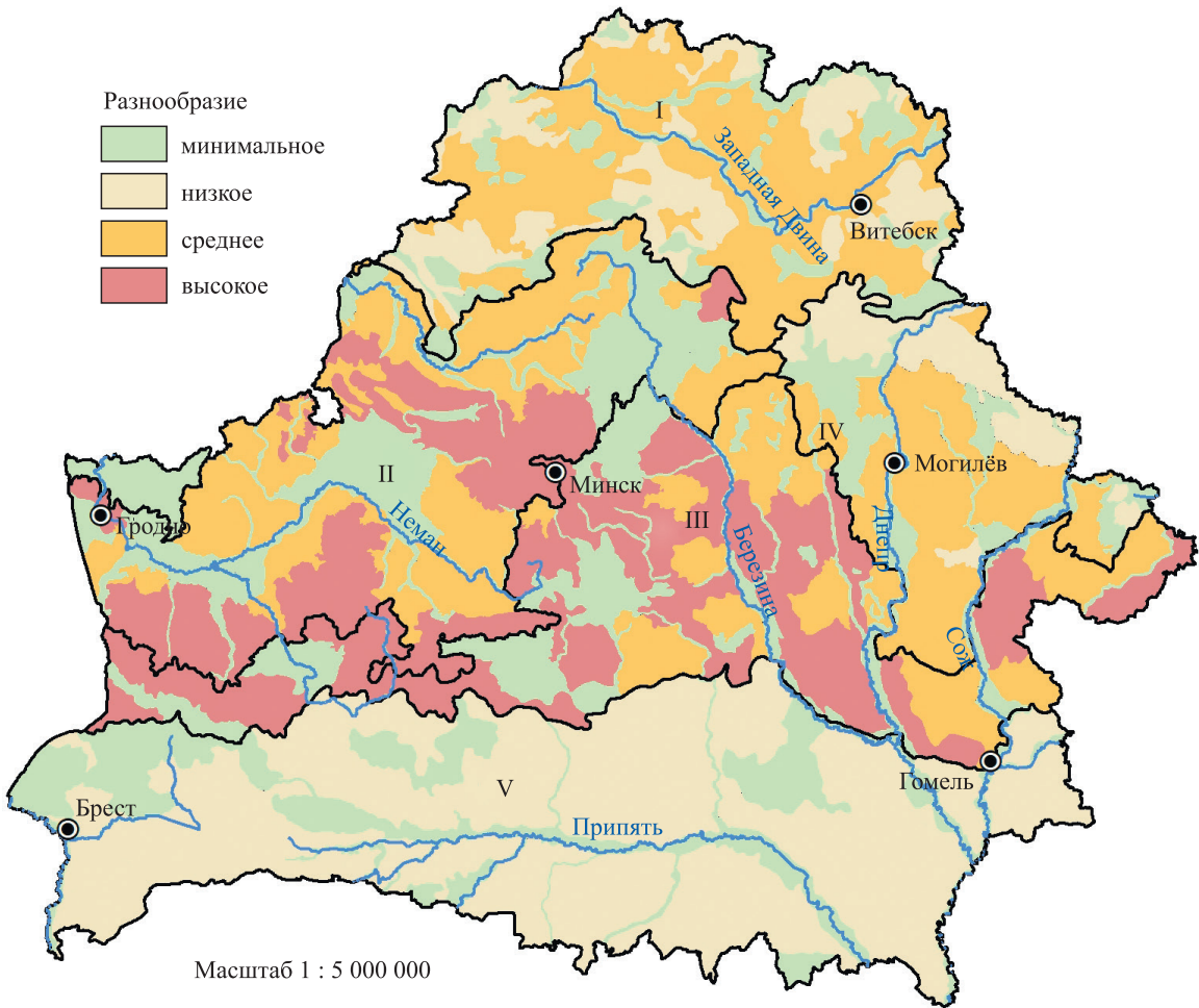
Рис. 2. Оценка ландшафтного разнообразия на уровне родов в разрезе провинций. Ландшафтные провинции: I – Поозерская; II – Белорусская возвышенная; III – Предполеская; IV – Восточно-Белорусская; V – Полеская
