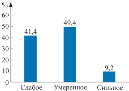
Рис. 3. Удельный вес случаев обледенения воздушных судов (2014–2018)
