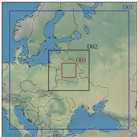
Рис. 1. Карта расположения ДМРЛ (а) и области моделирования в эксперименте с шагом сетки 9 км (D01), 3 км (D02), 1 км (D03) (б)
