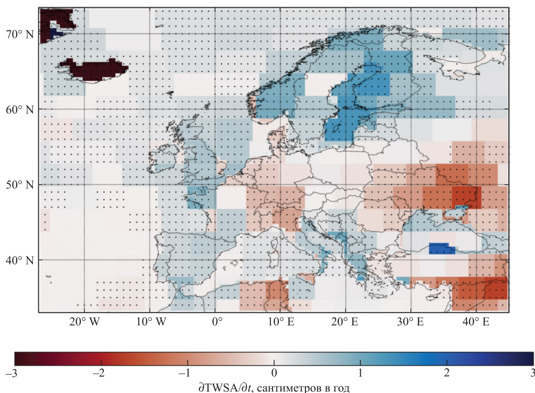
Рис. 4. Тренды изменений значений параметра TWSA для Европы за 2002–2017 гг. (точками отмечены области со статистически значимыми изменениями TWSA).
