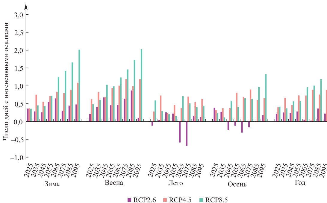
Рис. 7. Медианные оценки изменения числа дней с осадками, соответствующих 95-му процентилю, на территории Беларуси по ансамблю климатических моделей проекта EURO-CORDEX (EUR-11) за последовательные десятилетия в период 2021–2099 гг.
